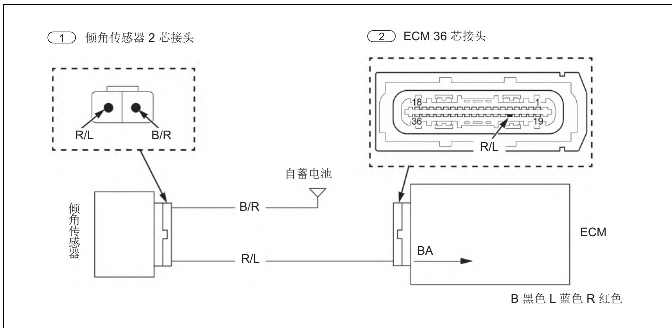
倾角传感器图
