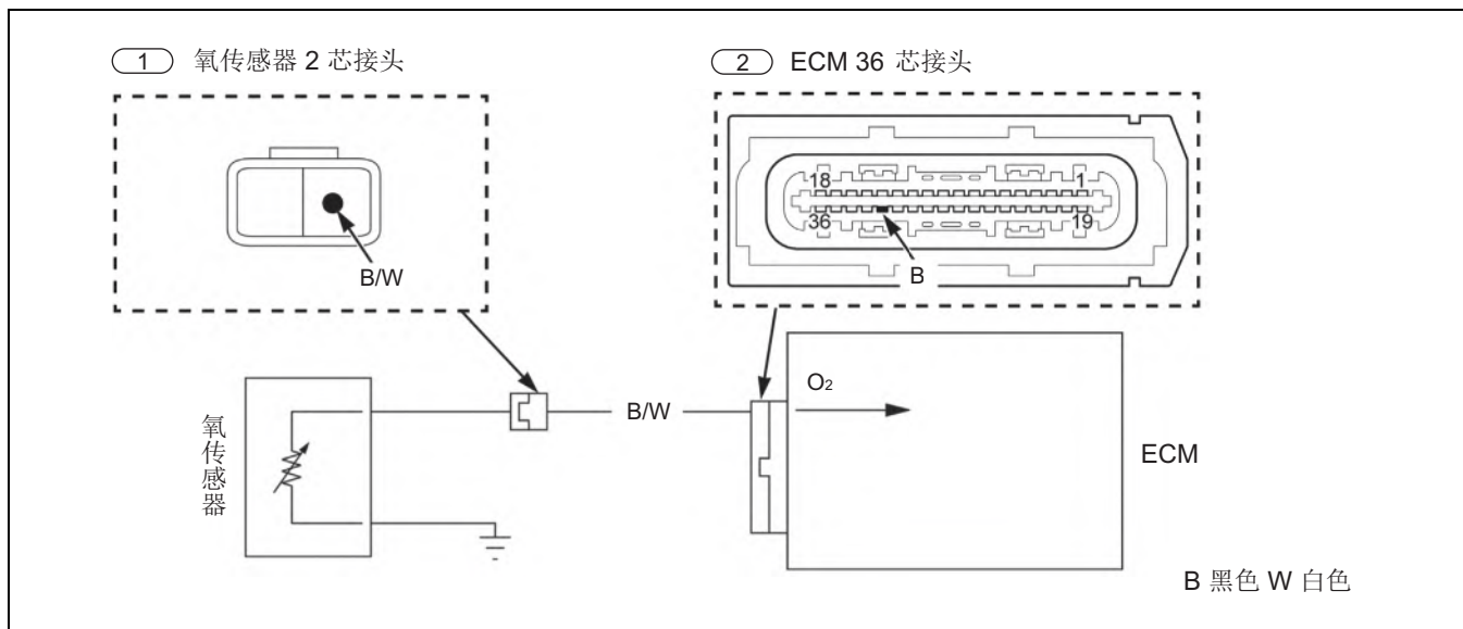
氧传感器图
