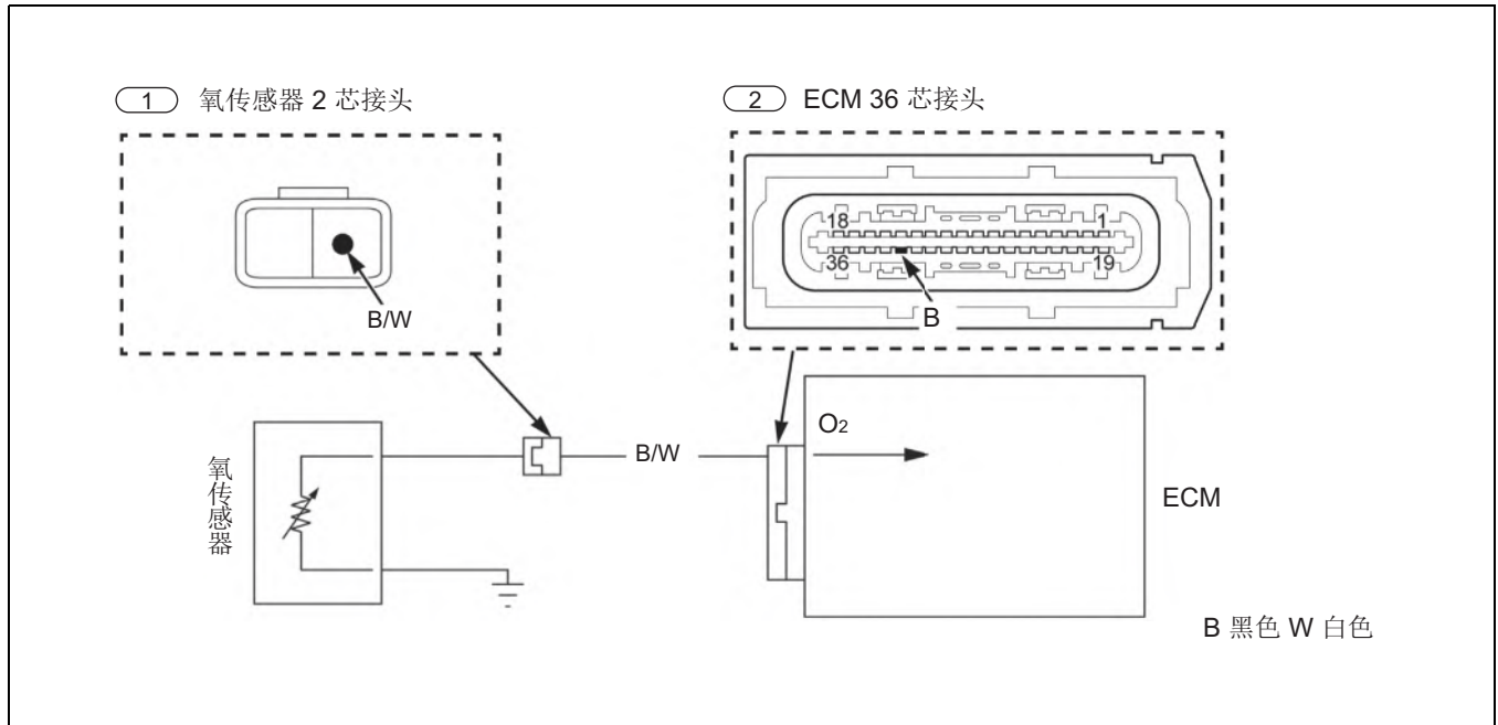
氧传感器图
