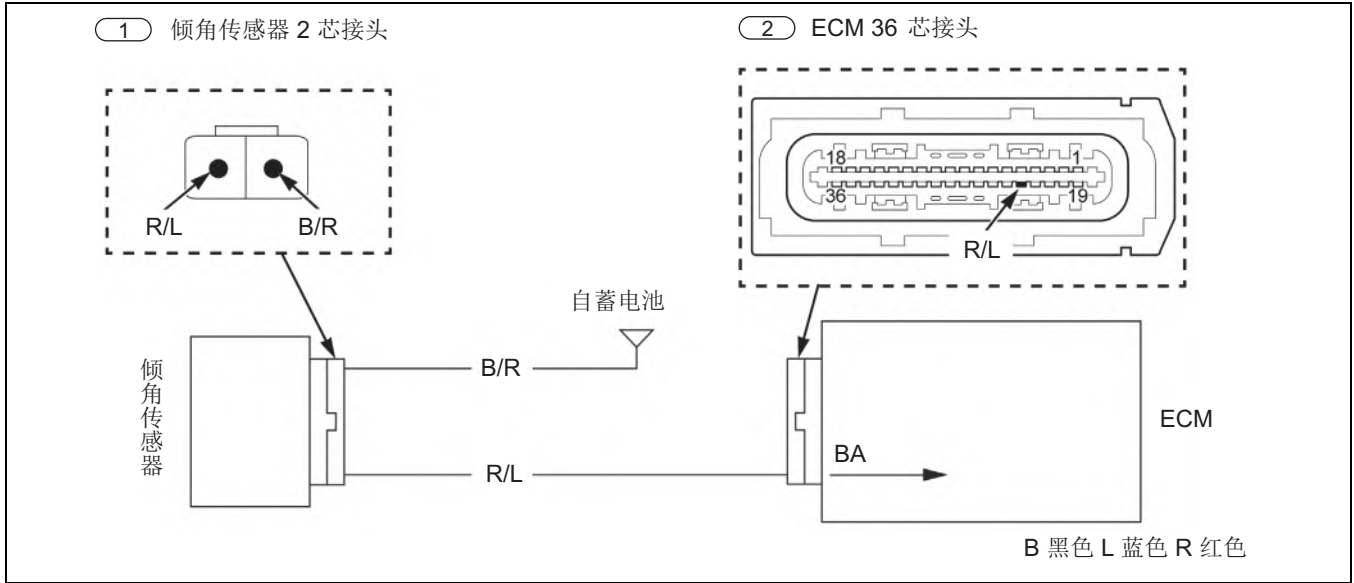
倾角传感器图
