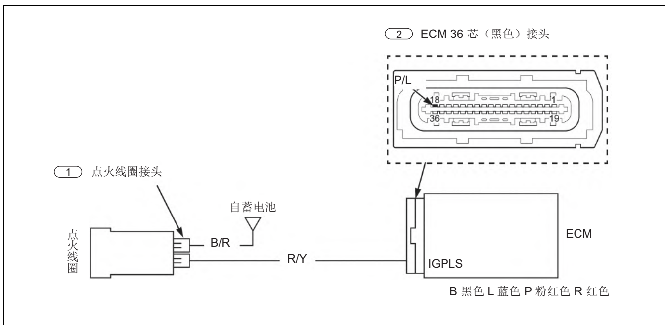
点火线圈初级电路图
