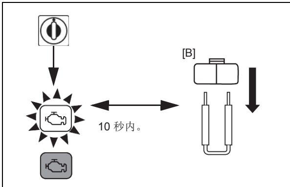
初始化步骤和 MIL 闪烁模式
