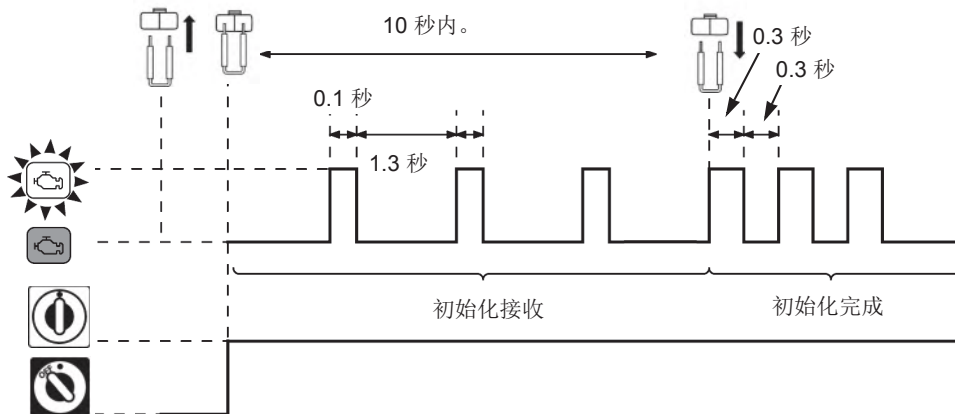
初始化步骤和 MIL 闪烁模式
